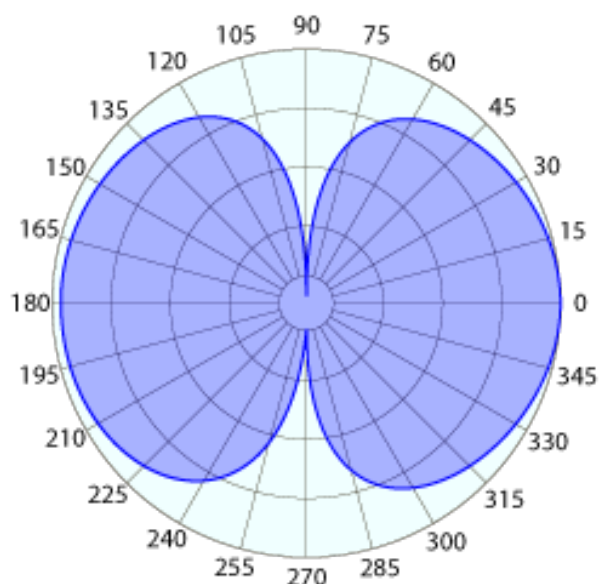
Вертикальная плоскость
